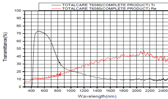
トータルケア U4-6580 分光曲線 黒色=透過率 赤色=反射率 紫外線400nmまで99.9%カット、赤外線 1000～1100nmで、81.6%カット
